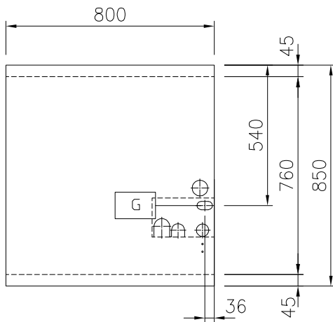
Boven aanzicht
