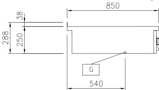
Zij aanzicht
